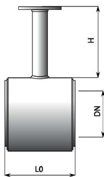
BEZPŘÍRUBOVÉ ČIDLO
