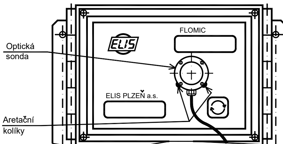
Obr. 40 - Umístění optické sondy
