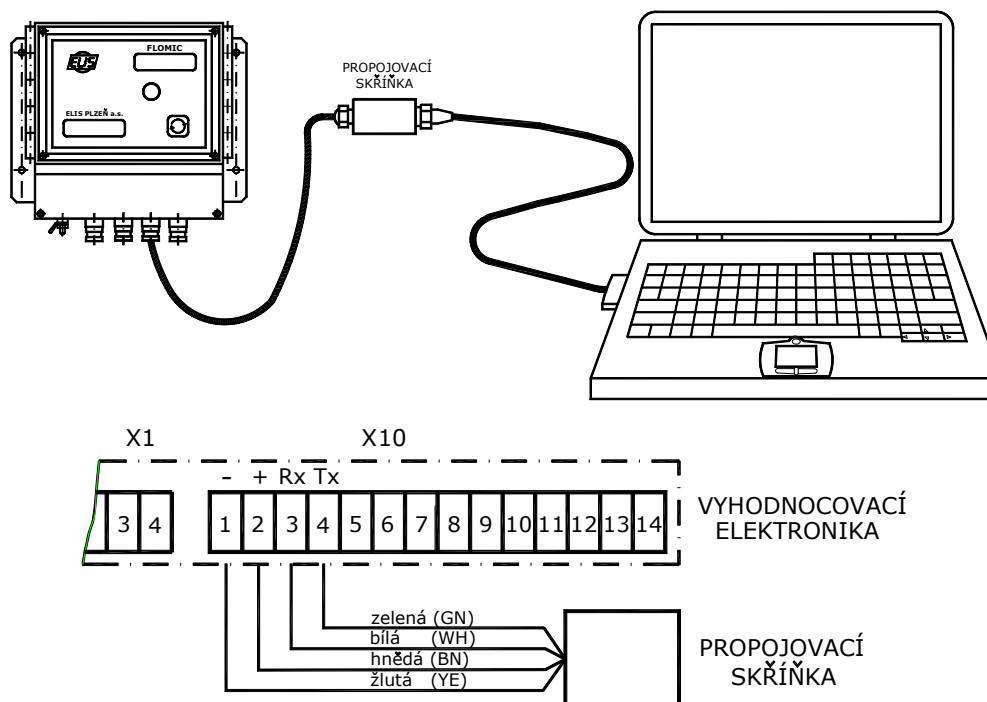
Obr. 42 - Komunikace přes linku RS 232
