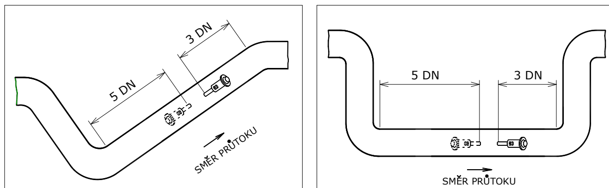
Obr. 16 - Umístění v dolní kapse
