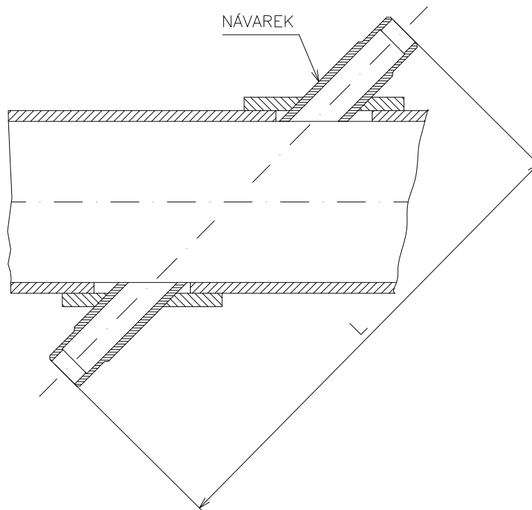
Obr. 29 - Určení vzdálenosti L
