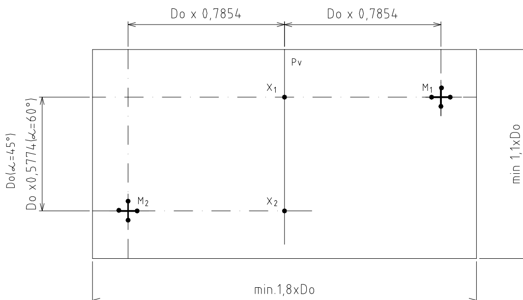
Obr. 23 - Papírová šablona
