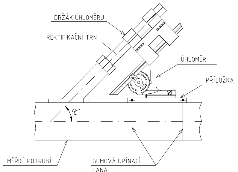
Obr. 28 - Stanovení úhlu měřicího paprsku
