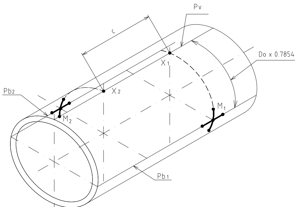
Obr. 22 - Rozměření montážních bodů
