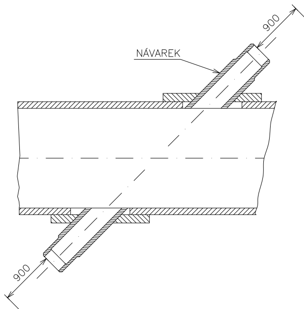
Obr. 20 - Volný prostor okolo návarek
