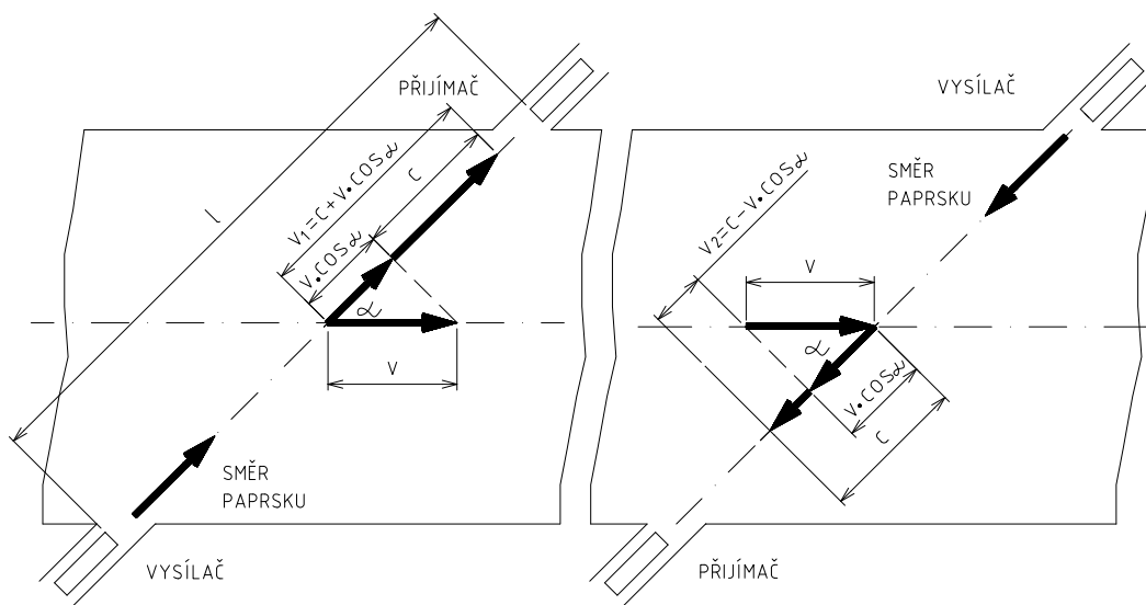
Obr. 1 - Princip činnosti
