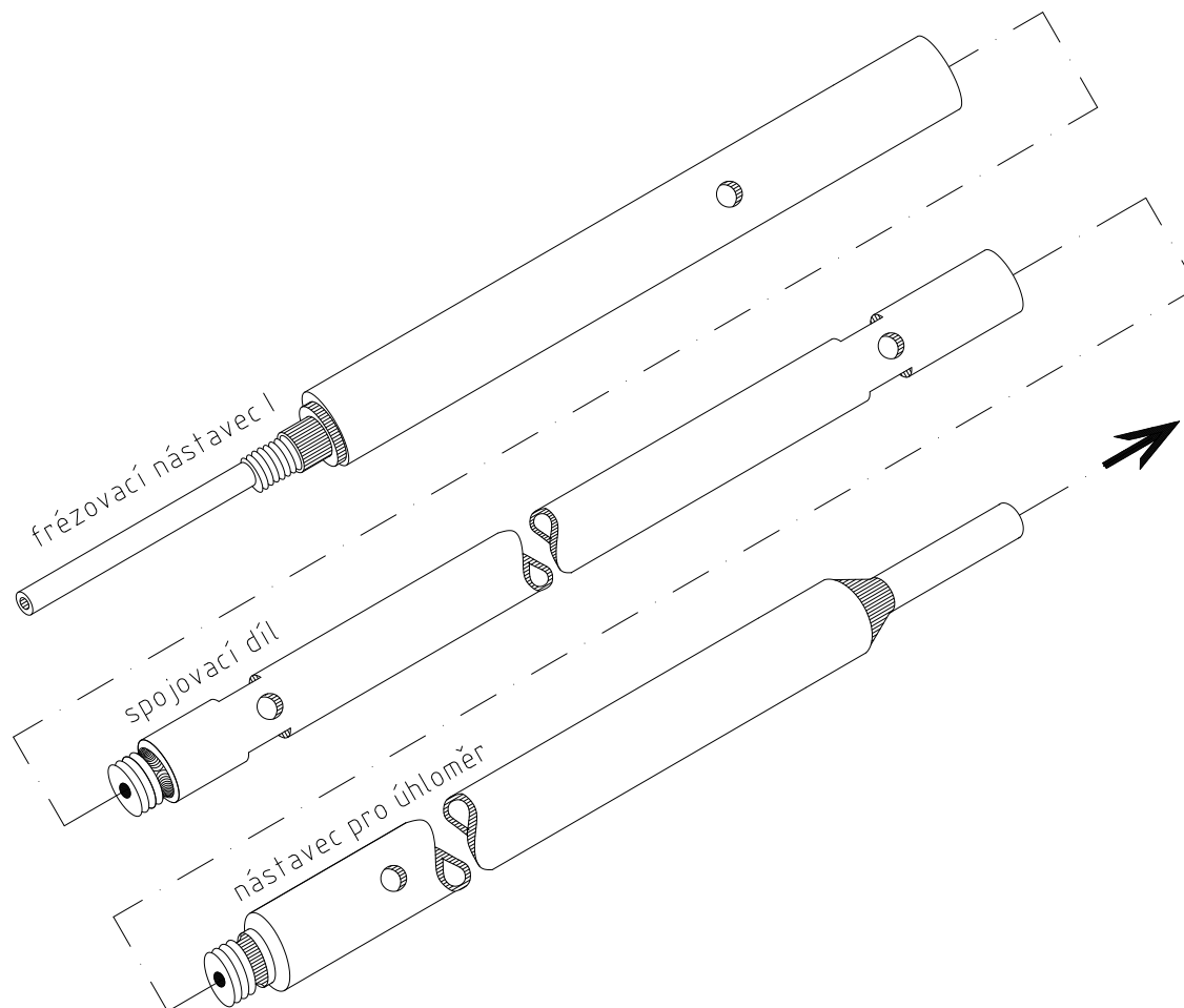
Obr. 25 - Sestavený rektifikační trn
