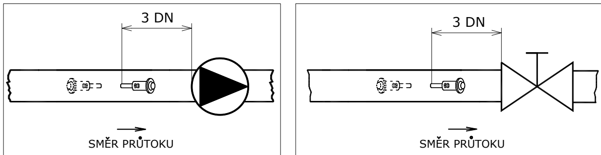
Obr. 15 - Uklidňující délky pro „poruchu“ za čidlem
