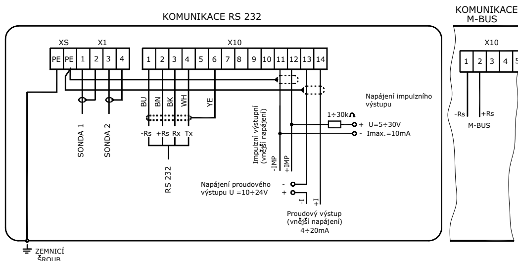
Obr. 30 - Zapojení signálových vstupů a výstupů elektroniky UP 8.00
