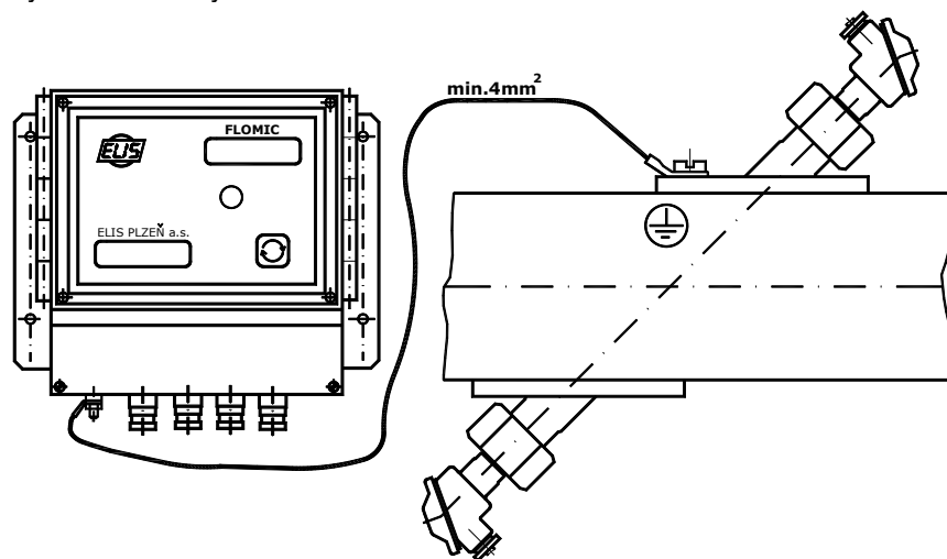
Obr. 19 - Připojení zemnění na skříňku elektroniky
