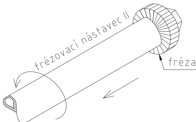
Obr. 27 - Zarovnání dosedací plochy nepřístupného návarku
