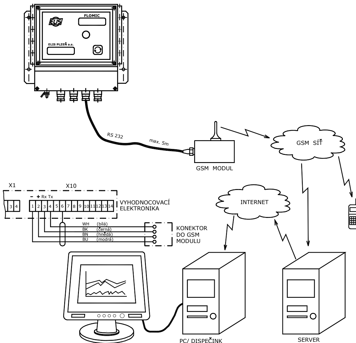
Obr. 43 - Odesílání dat z průtokoměru přes GSM bránu
