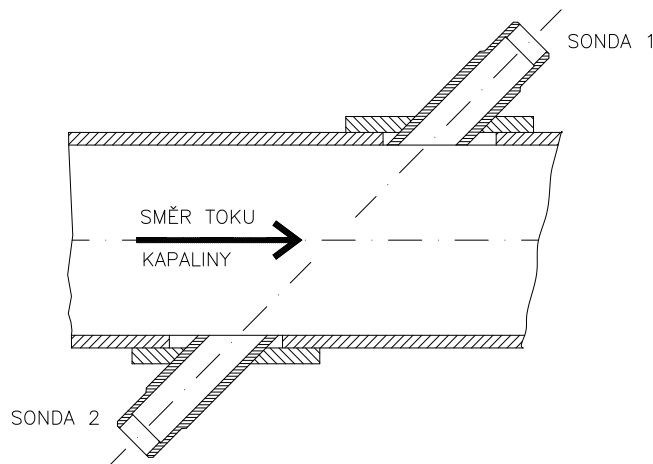
Obr. 31 - Označení sond
