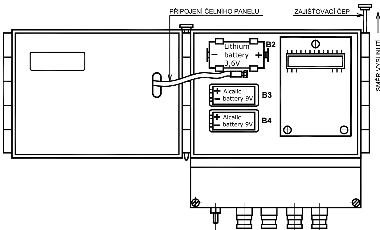
Obr. 44 - Výměna baterií
