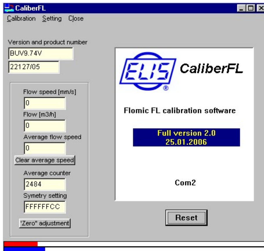
Obr. 37 - Kontrola nastavení nuly
