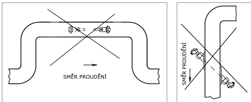
Obr. 18 - Nesprávné umístění čidla
