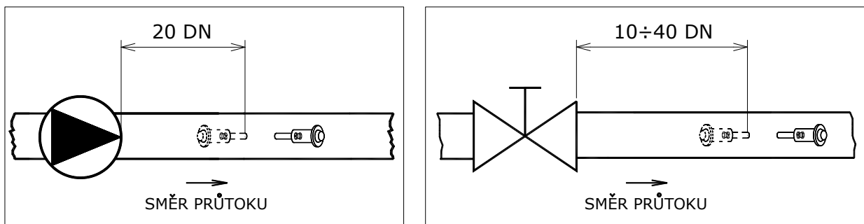
Obr. 14 - Uklidňující délky pro „rušivé vlivy“ před čidlem
