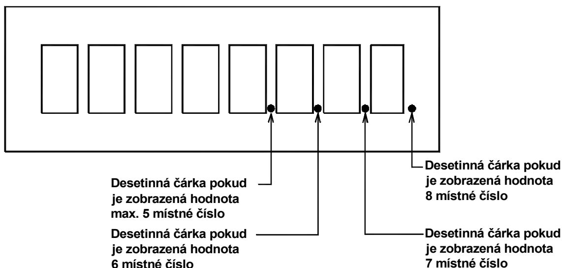
Obr. 15 - Umístění desetinných čárek na displeji
