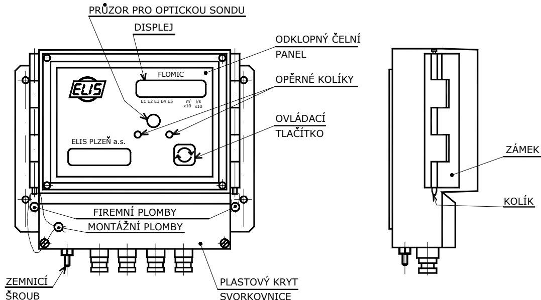
Obr. 4 - Vyhodnocovací elektronika – popis
