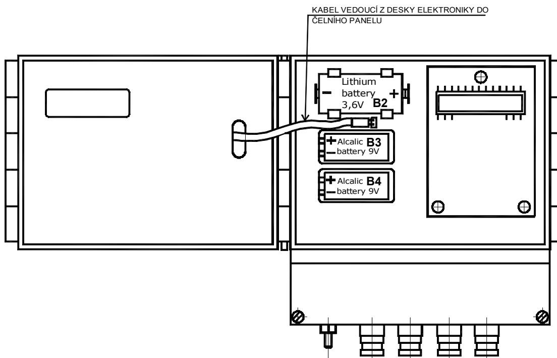
Obr. 20 - Výměna baterií
