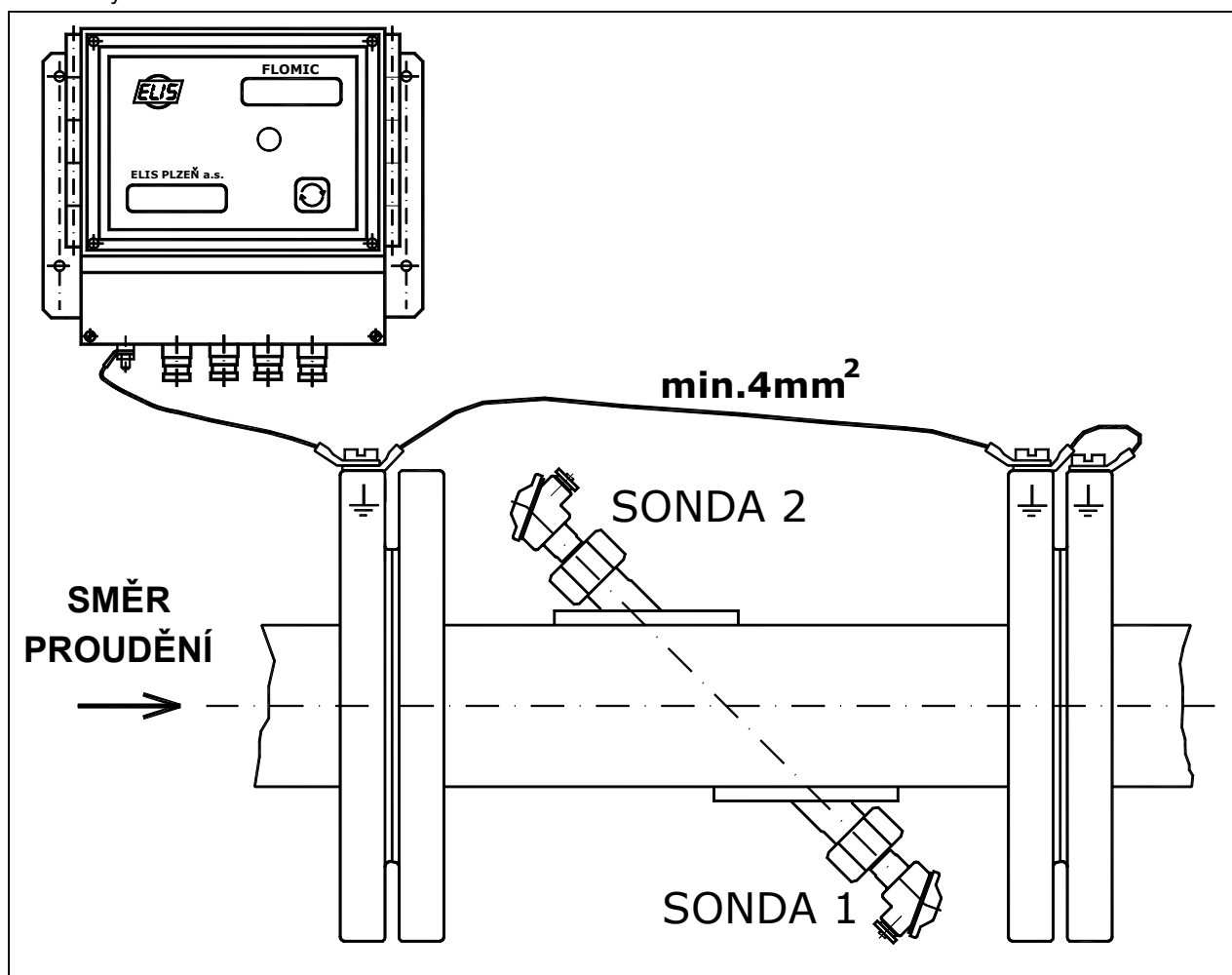
Obr. 13 - Uzemnění elektroniky a čidla průtokoměru
