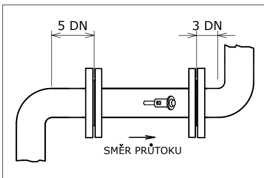
Obr. 6 - Minimální uklidňující délky
