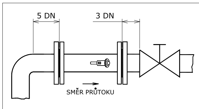
Obr. 7 - Minimální délka před uzavíracím kohoutem
