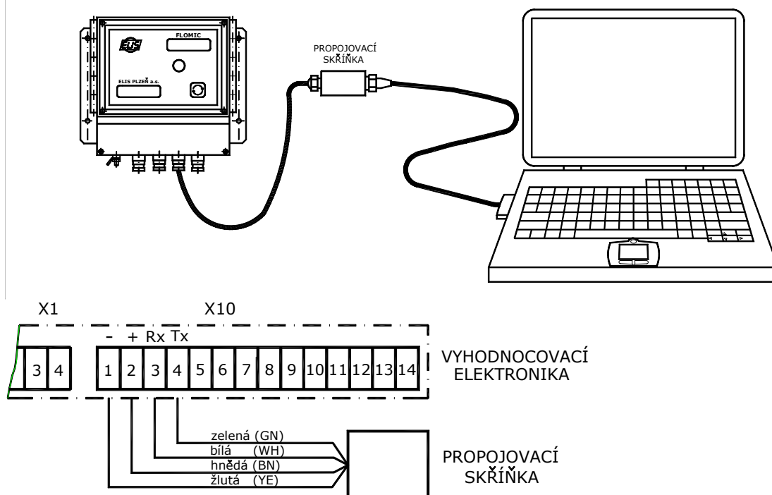
Obr. 18 - Komunikace přes linku RS 232
