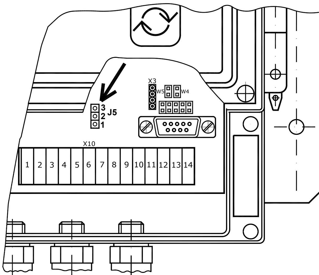
Obr. 16 - Změna nastavení doby trvání impulsu propojkou J5
