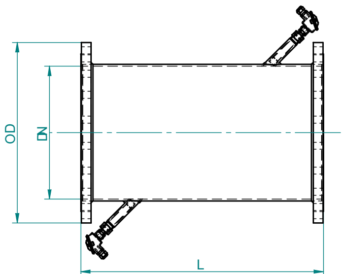
Obr. 1 - Rozměrový náčrt čidla
