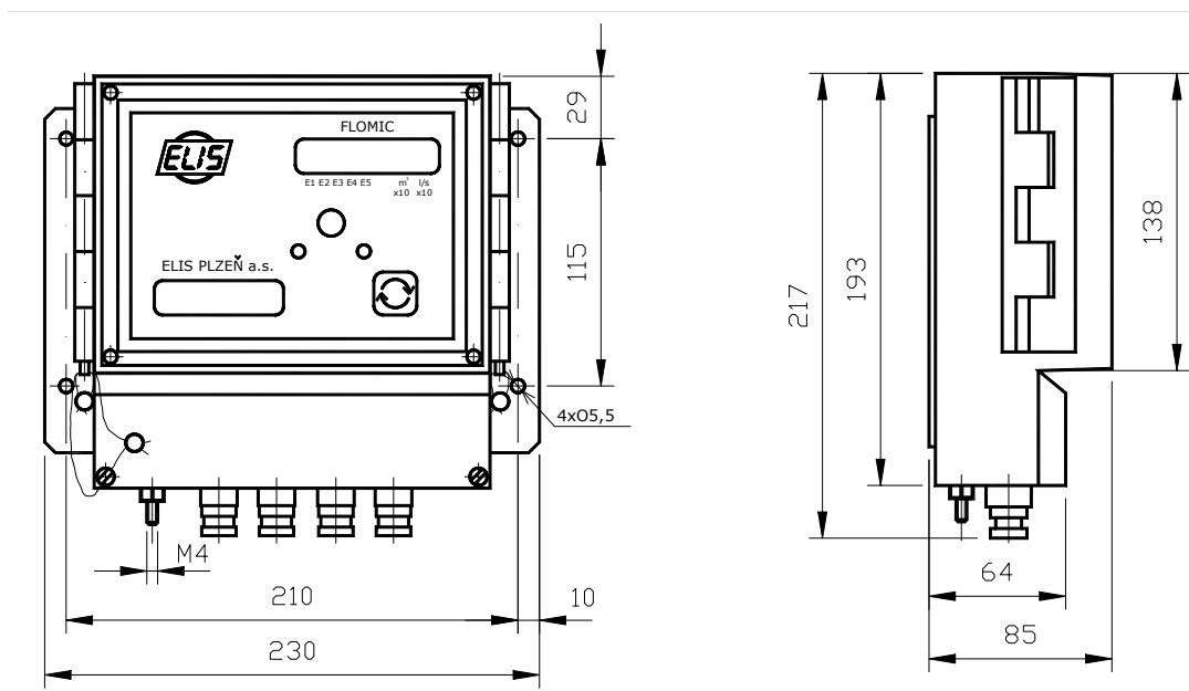
Obr. 2 - Rozměrový náčrt skříňky elektroniky
