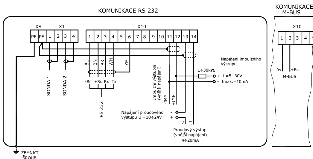
Obr. 14 - Elektrické připojení
