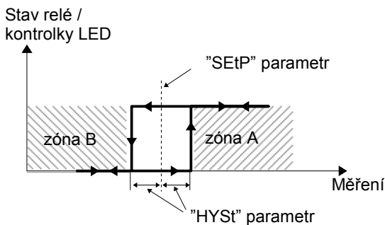
Obrázek 6.4. Jednopráhové řízení releových výstupů a kontrolkek LED R1÷R4
